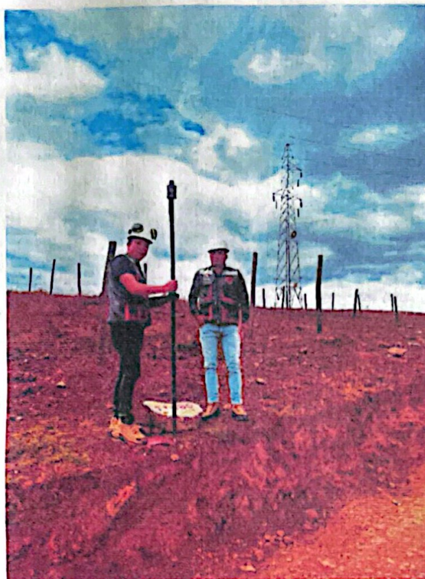
FOTOGRAFIA N° 17 : SE MUESTRA LA VERIFICACIÓN CORTE A 50 CM DESDE LA SEÑALIZACIÓN DEL REPLANTEO.
