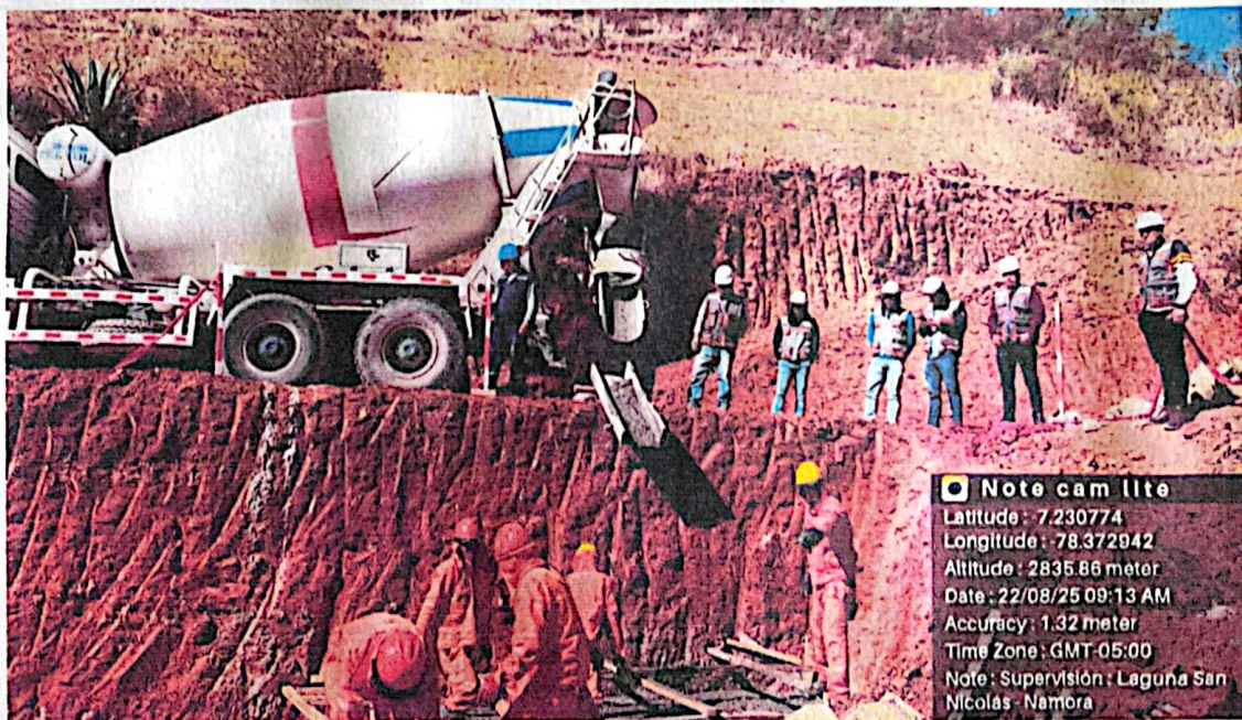
FOTOGRAFIA N° 12 : SE MUESTRA LA VERIFICACION EN EL VACIADO DE ZAPATAS, EN LOS MUROS DE CONTECCION.
