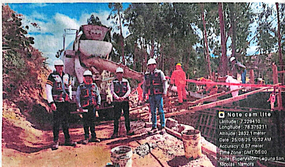
FOTOGRAFIA N° 04: SE MUESTRA EL LA VERIFICACIÓN DEL VACIADO DE CONCRETO CICLOPEO EN ZAPATAS DE MURO f'c = 175 \text{ Kg/Cm}^2
