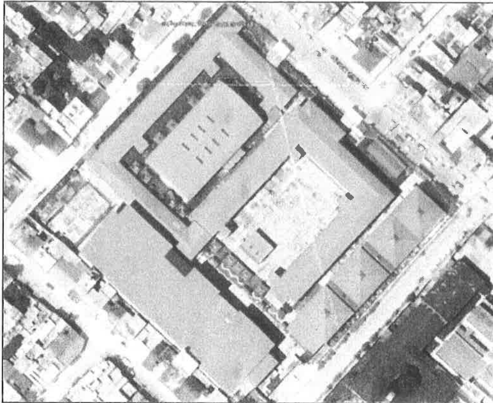
Imagen satelital actual I.E. Emblemático Santa Teresita – Distrito Cajamarca CAJAMARCA – 2023. Fuente: Elaboración propia.
